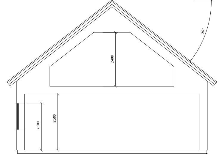
Sektion
