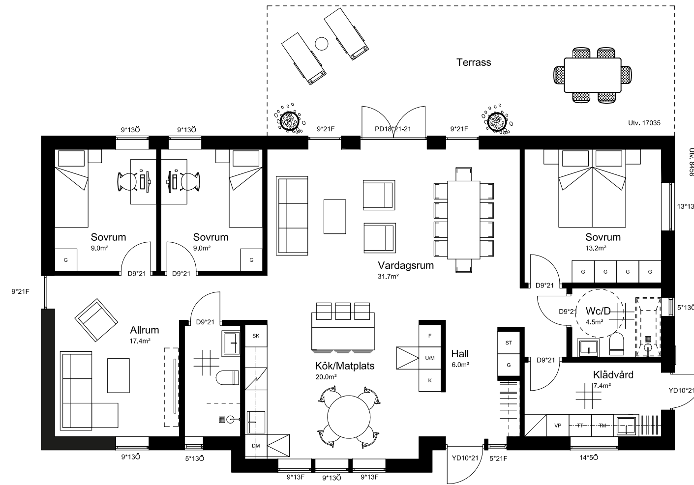
Planlösning BOA/Inv. yta 129m 2
